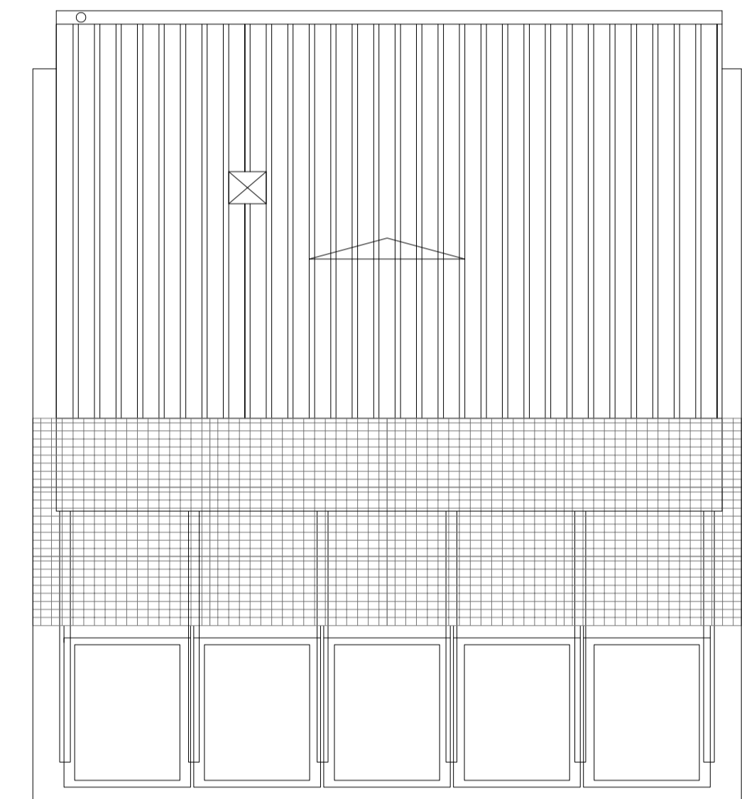
PLANTA COBERTES COTXERIA/SALA DE MÀQUINES
