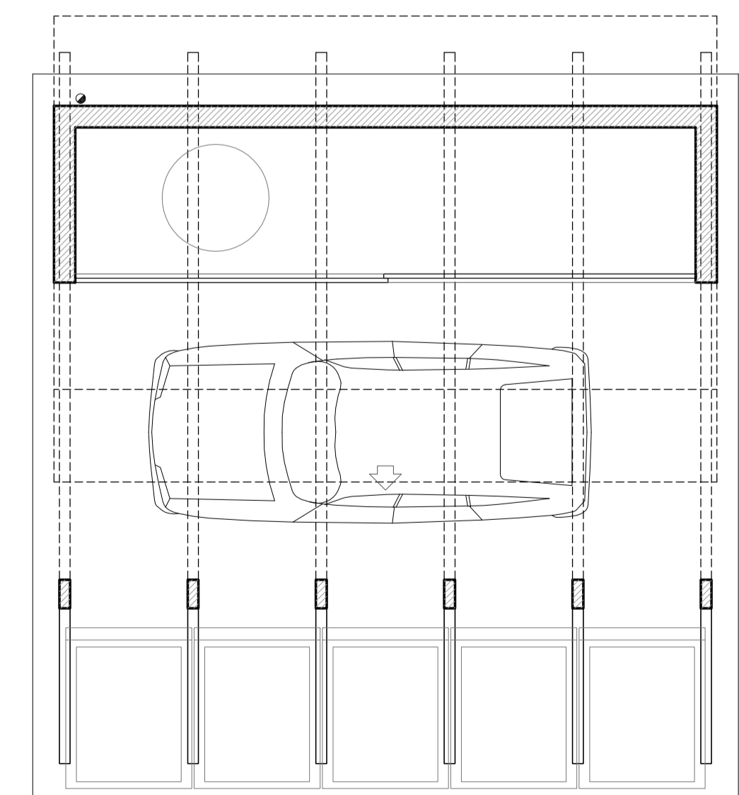
PLANTA BAIXA COTXERIA/SALA DE MÀQUINES
