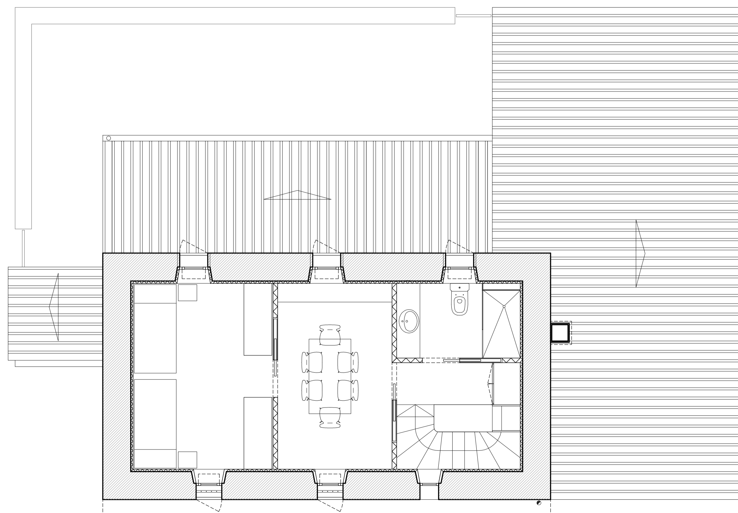
PLANTA PIS VIVENDA
