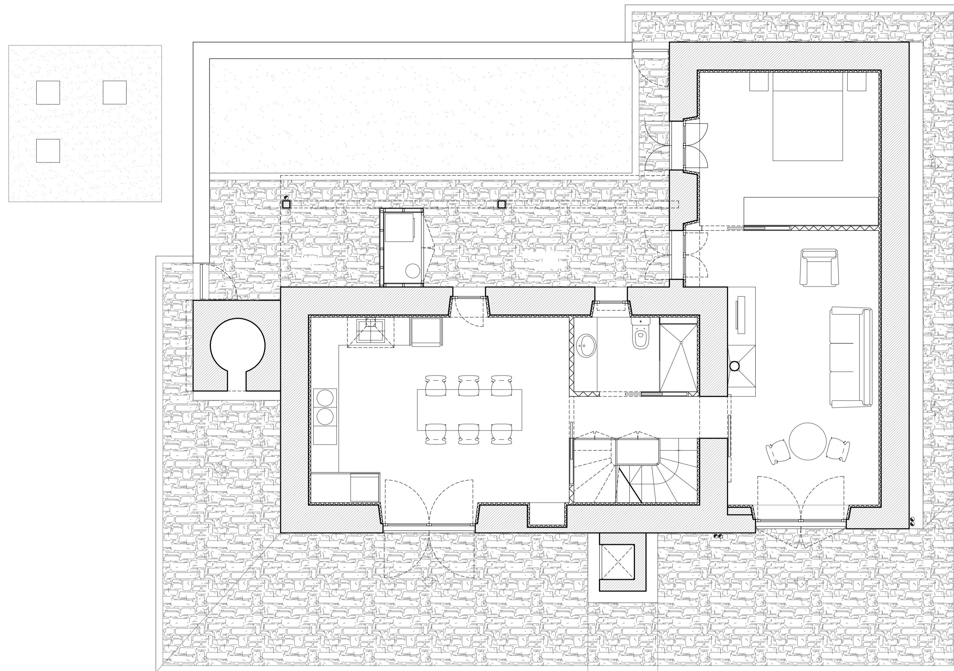
PLANTA BAIXA VIVENDA
