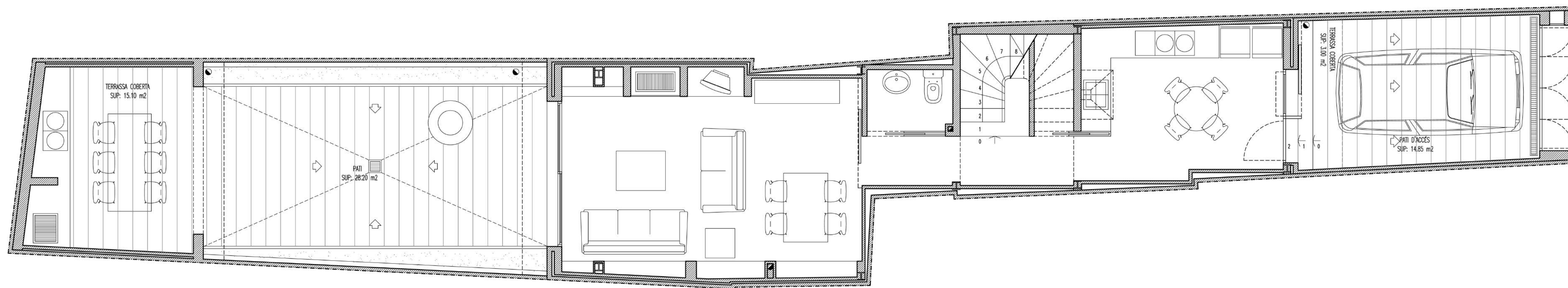
PLANTA BAIXA
