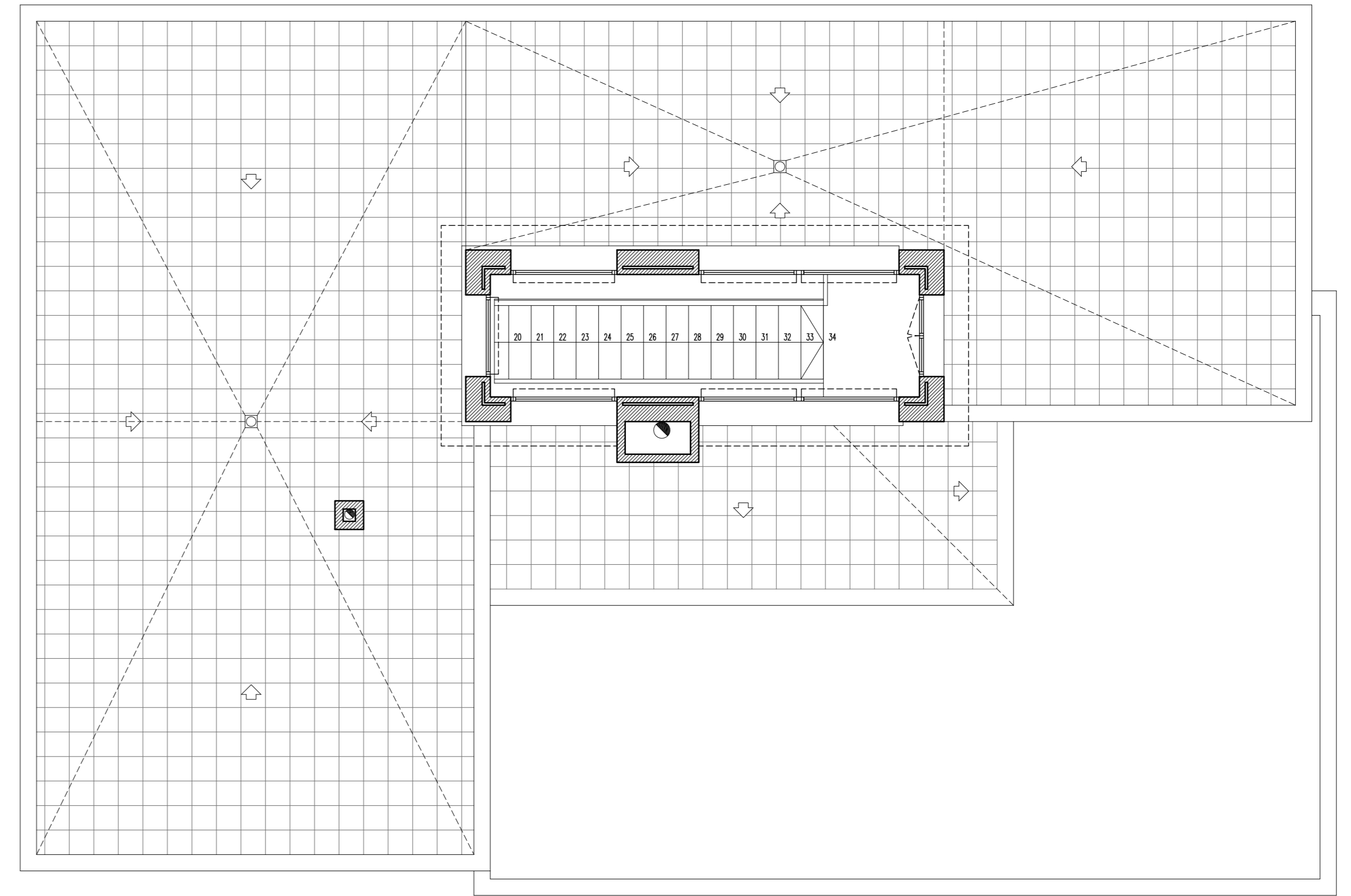
PLANTA COBERTA
