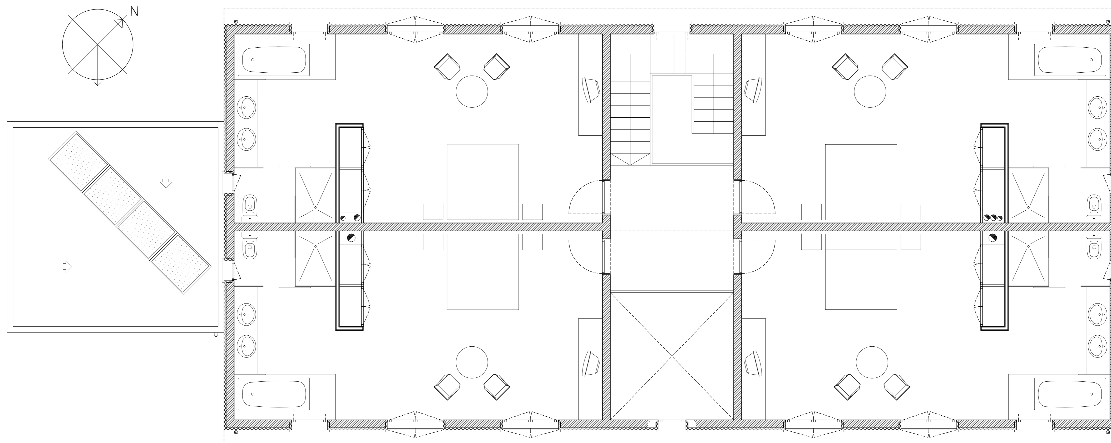
PLANTA PRIMERA
