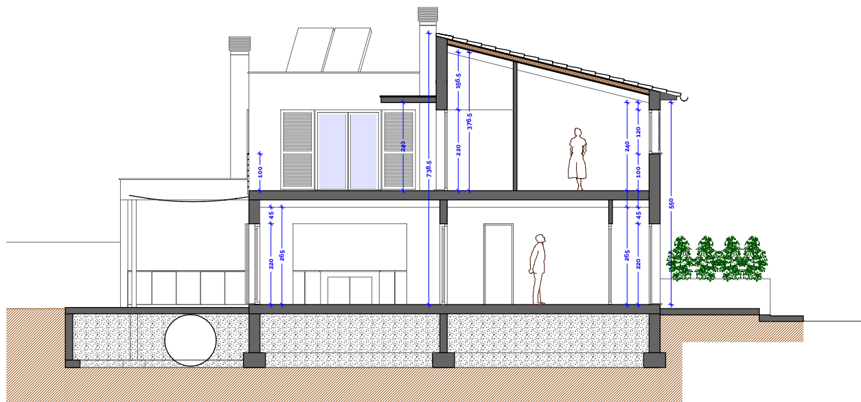
S1 - SECCIÓ PER ENTRADA I SALA-MENJADOR
