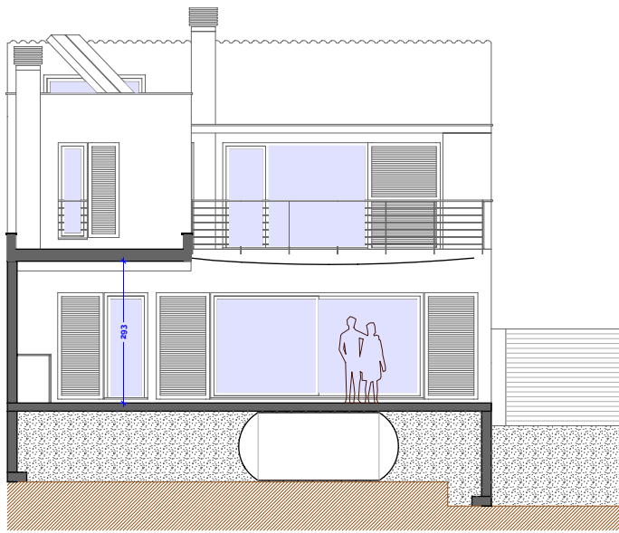
S2 - SECCIÓ PER TERRASSA PB
