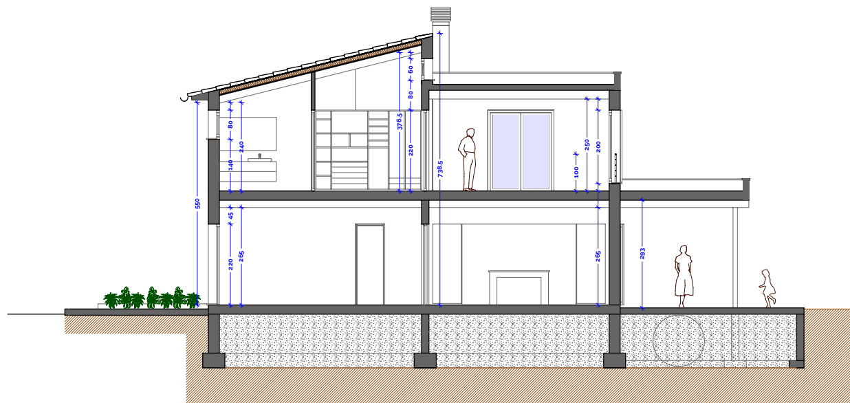
S4 - SECCIÓ PER CUINA I HABITACIÓ PRINCIPAL
