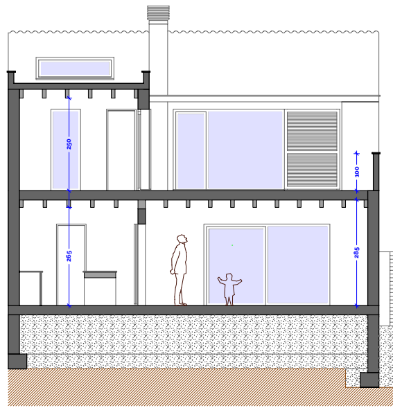
S3 - SECCIÓ PER TERRASSA PPIS
