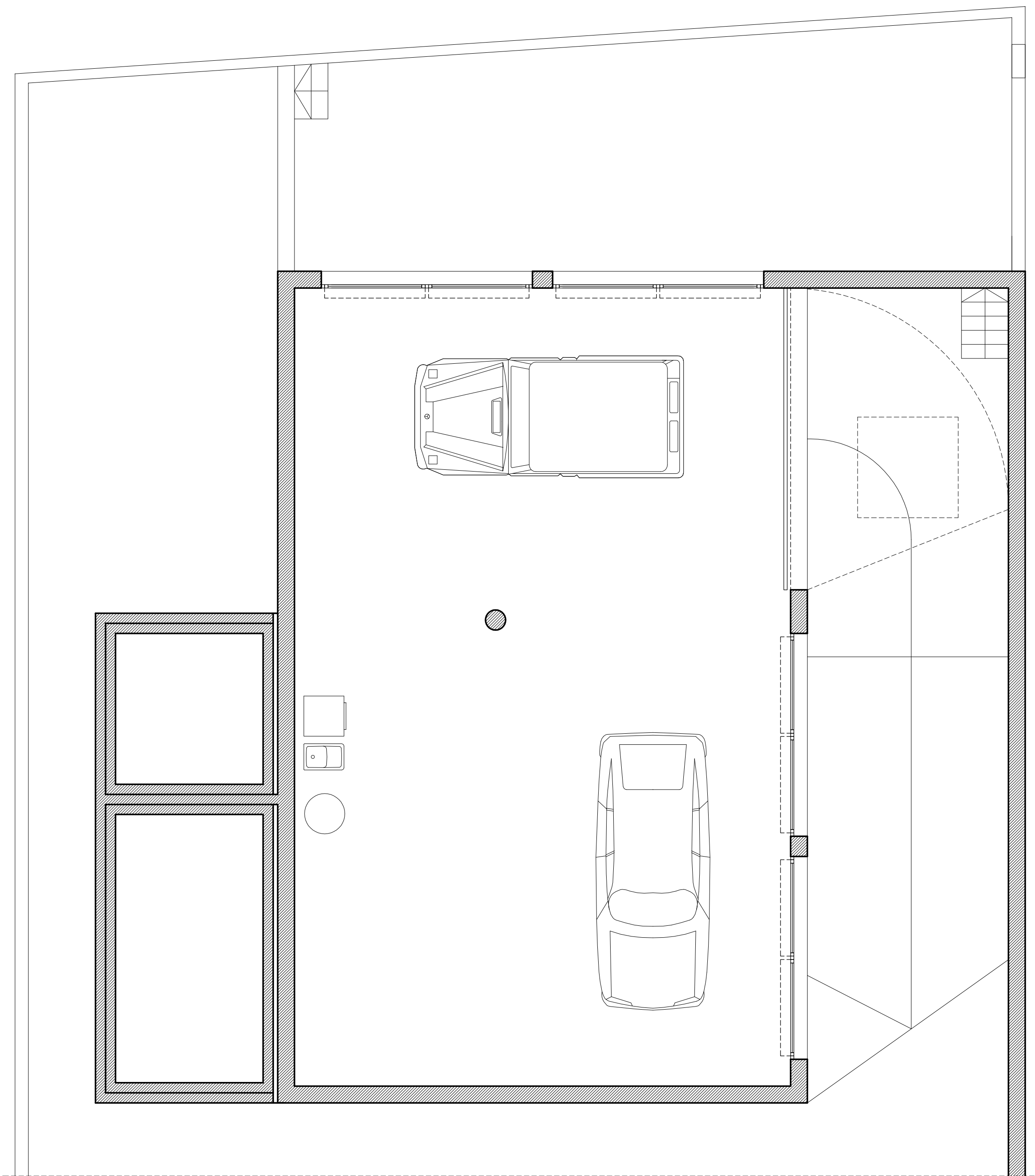
PLANTA SOTERRANI
