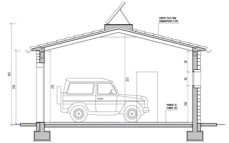
S1 - SECCIÓ TRANSVERSAL DE COTXERIA
