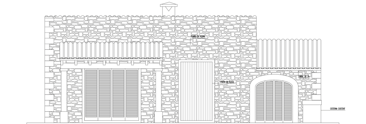
F1 - FAÇANA PRINCIPAL
