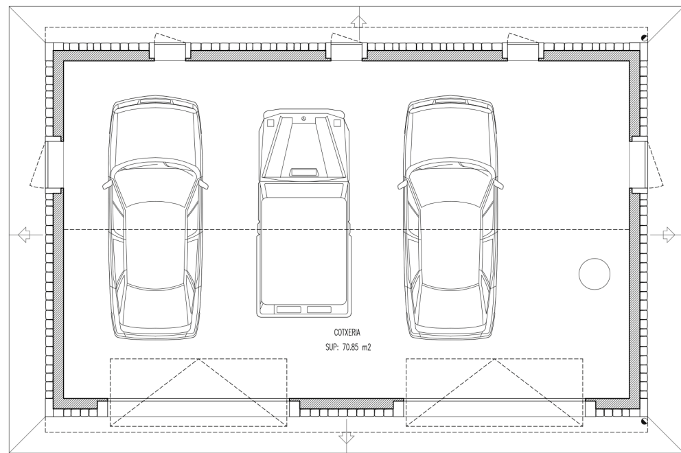
COTXERIA PLANTA BAIXA
