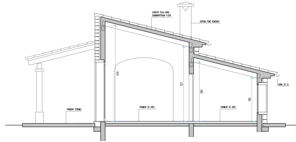
S2 - SECCIÓ PER SALA-HABITACIÓ (ZONA REFORMADA)
