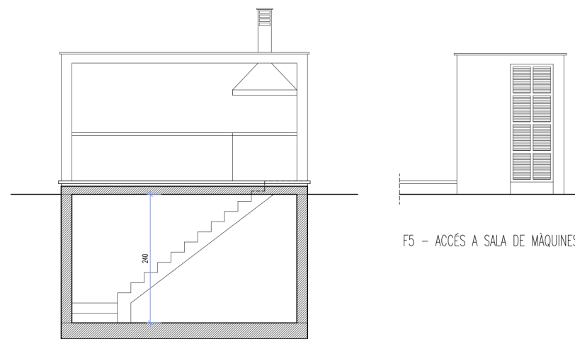
S3 - SECCIÓ TRANSVERSAL DE SALA DE MÀQUINES
