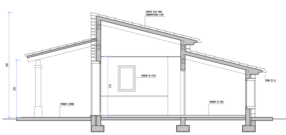
S1 - SECCIÓ PER PORXO-CUINA-BANY (ZONA AMPLIADA)
