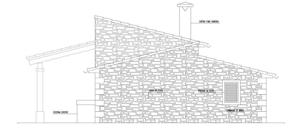
F2 - FAÇANA LATERAL DRETA
