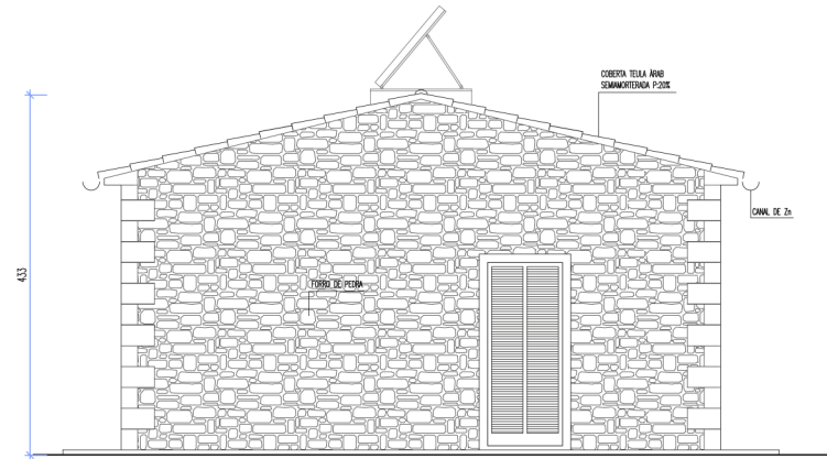
F2 - FAÇANA LATERAL DRETA
