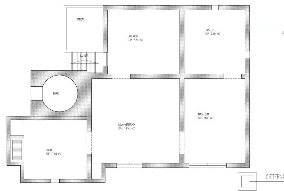
PLANTA BAIXA E:1/50
