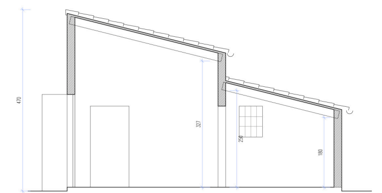
S1 - SECCIÓ PER SALA-MENJADOR-HABITACIÓ
