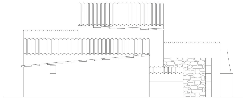
F2 - FAÇANA POSTERIOR
