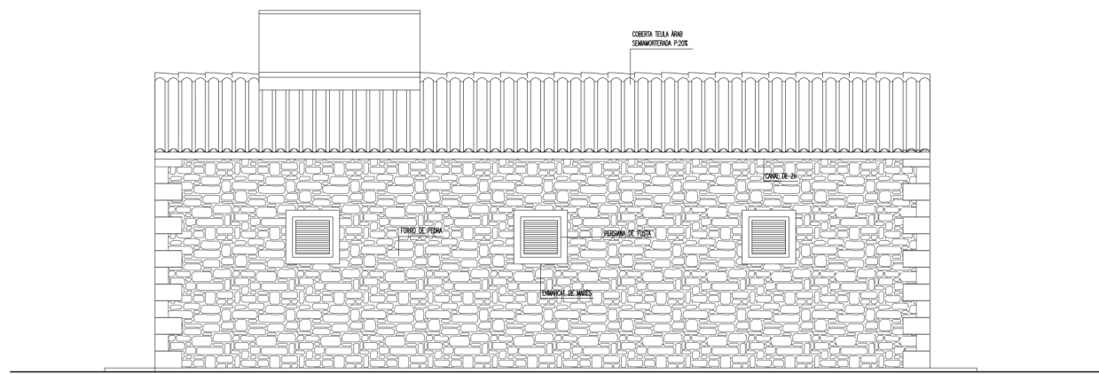
F3 - FAÇANA POSTERIOR
