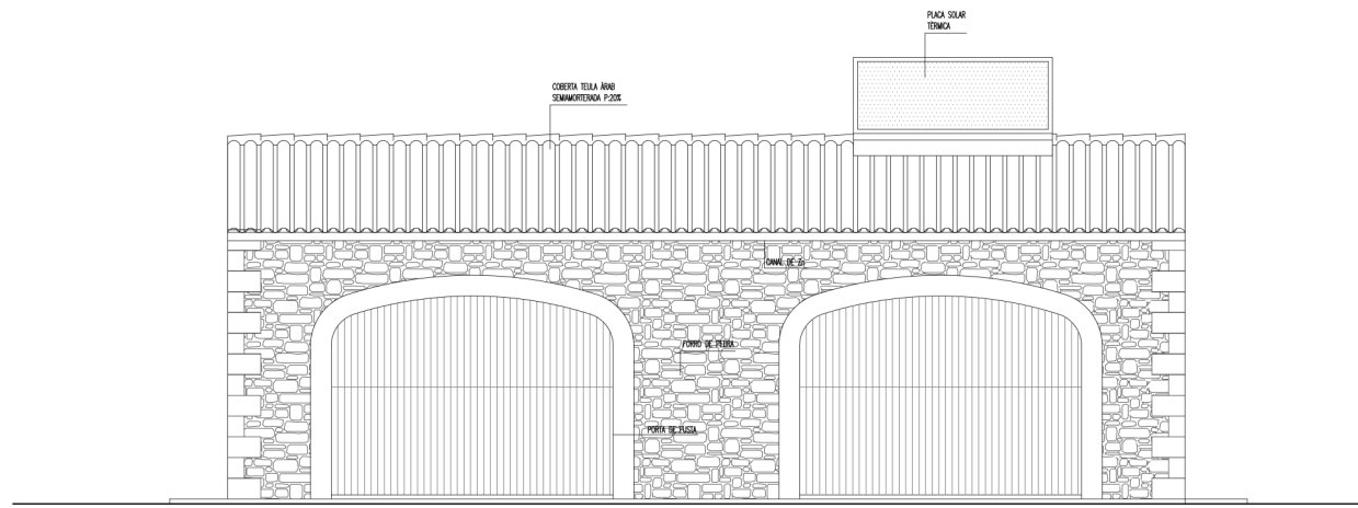
F1 - FAÇANA PRINCIPAL
