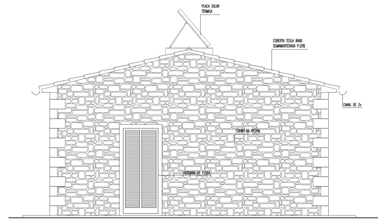
F4 - FAÇANA LATERAL ESQUERRA
