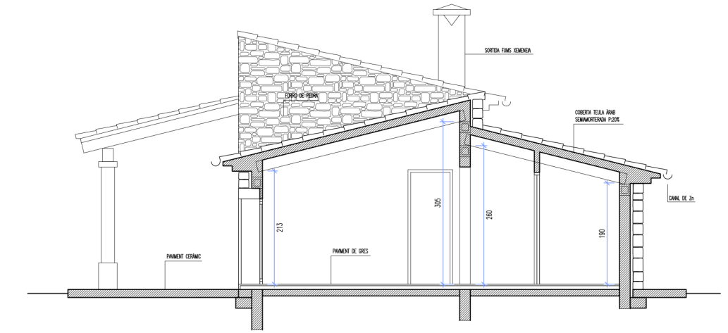
S3 - SECCIÓ PER HABITACIÓ-BANY (ZONA REFORMADA)
