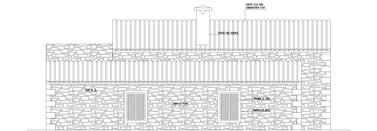
F3 - FAÇANA POSTERIOR
