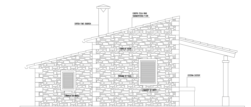
F4 - FAÇANA LATERAL ESQUERRA
