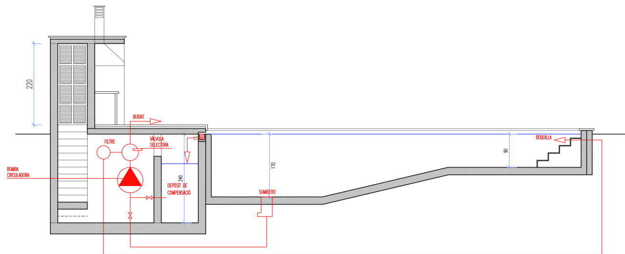
S2 - SECCIÓ PER PISCINA I SALA DE MÀQUINES
